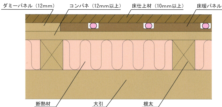
標準施工断面図
