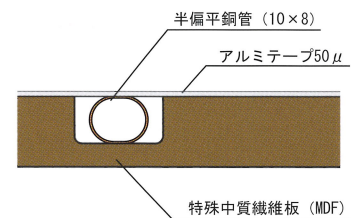
断面図
